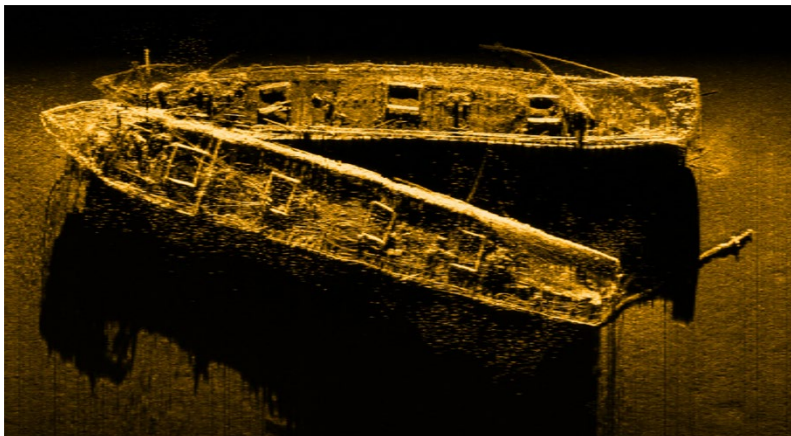
4K-SVY - SS Frank A. Palmer & Louise B. Cary -Colliers Stellwagen Bank
